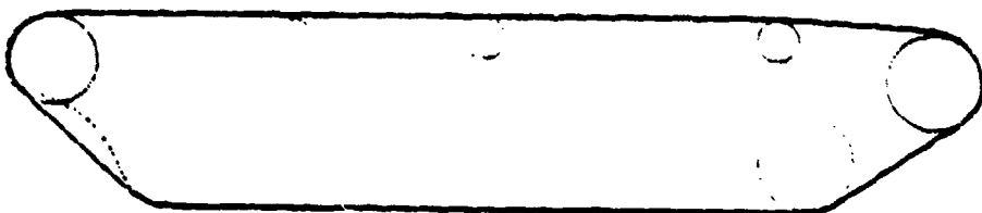
g. Seventh Mode, f = 8.806 Hz
