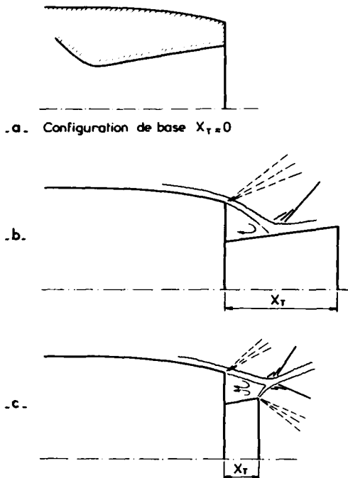
Fig. 38 EFFET D'EMERGENCE DE LA TUYERE
