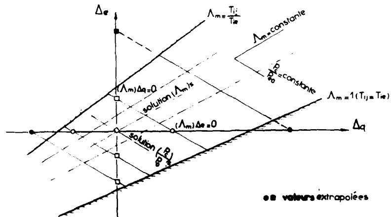
Fig. 92 RECHERCHE DE LA SOLUTION POUR LA PRESSION ET LA TEMPERATURE DE L'ECOULEMENT ISOENERGETIQUE ( d'ADDY )
