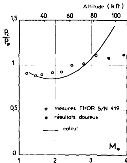
Fig. 100 PRESSION DE CULOT D'UN ENGIN MONOTUYERE COMPARAISON A DES MESURES EN VOL (Théorie de HONG [93])
