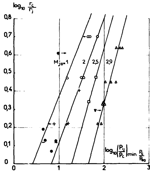
Fig. 39 CORRELATION POUR LA VALEUR MINIMALE DU RAPPORT \frac{P_c}{P_{e0}} (d'après [30])
