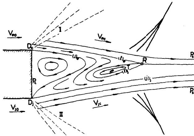
Fig. 34 SCHEMATISATION DE LA CONFLUENCE EN AVANT D'UN CULOT
