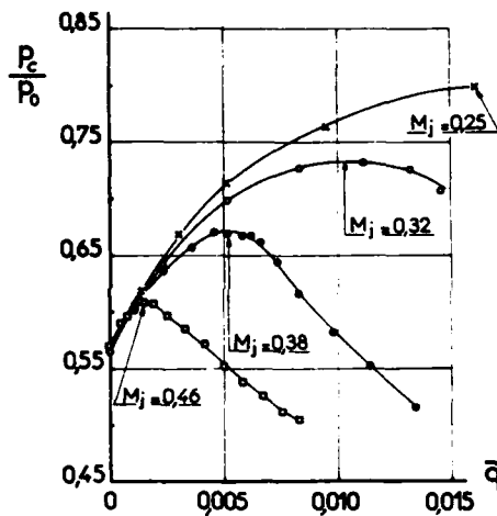
Fig. 30 EFFET DE VENTILATION SUR LA PRESSION DE CULOT ECOULEMENT EXTERNE SUPERSONIQUE (d'après [27])
