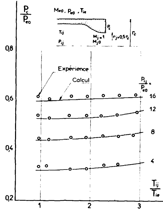
Fig 94 EFFETS THERMIQUES SUR LA PRESSION DE CULOT THEORIE D'ADDY
