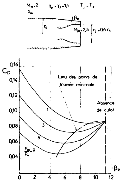
Fig. 99 OPTIMISATION DE LA TRAINEE TOTALE (culot+rétréint) D'UN ARRIERE CORPS (d'après ADDY [90])
