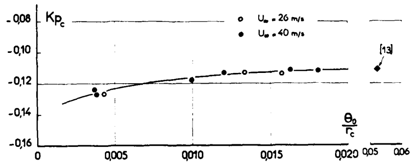
Fig. 6 EFFET DE COUCHE LIMITE INITIALE SUR LE COEFFICIENT DE PRESSION DE CULOT. ECOULEMENT INCOMPRESSIBLE (d'après [ 11 ])
