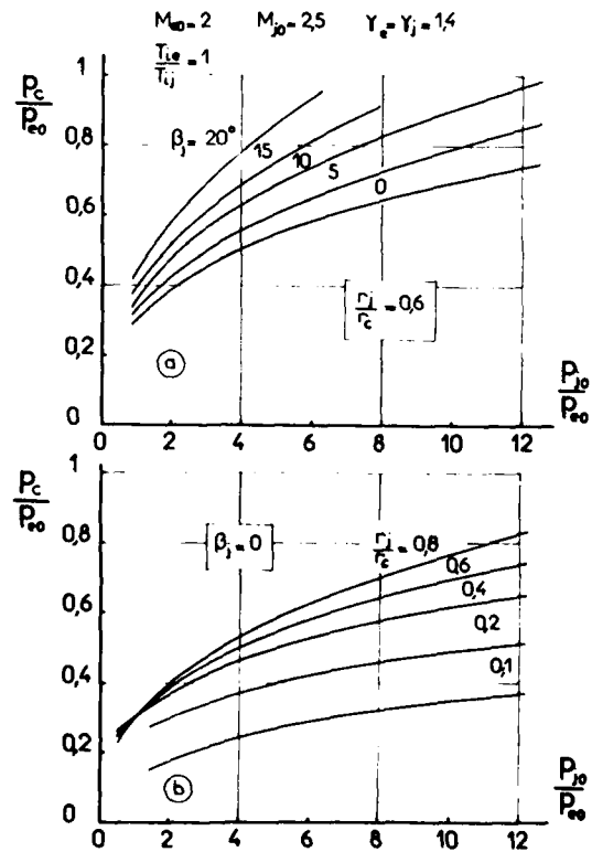
Fig. 96 VARIATION PARAMETRIQUE DES FACTEURS GEOMETRIQUES: DEMI-ANGLE DE LA TUYERE (a) RAYON DE LA TUYERE (b) (d'après ADDY [90])
