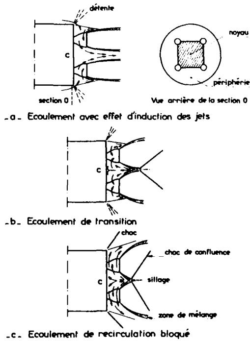
Fig. 46 STRUCTURE DE L'ECOULEMENT AU CULOT D'UN MISSILE QUADRITUYERES
