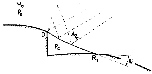
Fig 61- GENERALISATION DE LA NOTION D'ANGLE DE RECOLLEMENT
