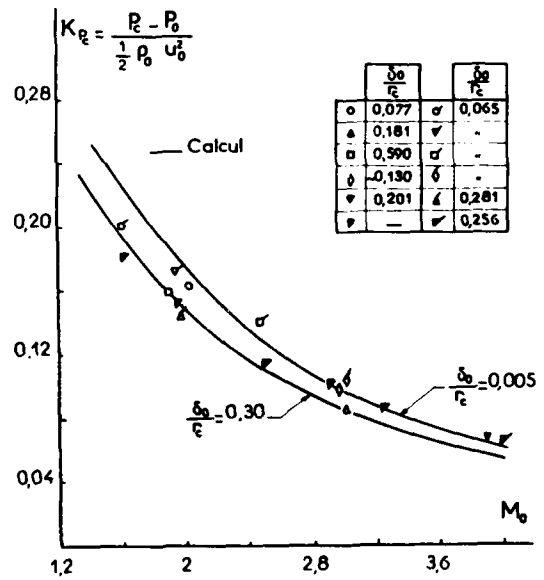
Fig. 75 - EFFET DU NOMBRE DE MACH AMONT SUR LA PRESSION DE CULOT (THEORIE de MEHTA)
