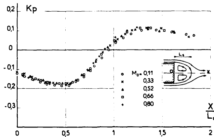
Fig. 9 EVOLUTION DU COEFFICIENT DE PRESSION SUR L'AXE ECOULEMENT SUBSONIQUE (d'après [ 13 ])
