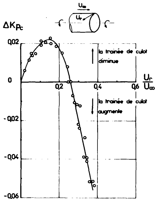
Fig. 29 EFFET DE ROTATION SUR LA PRESSION DE CULOT ECOULEMENT SUBSONIQUE (d'après [26])
