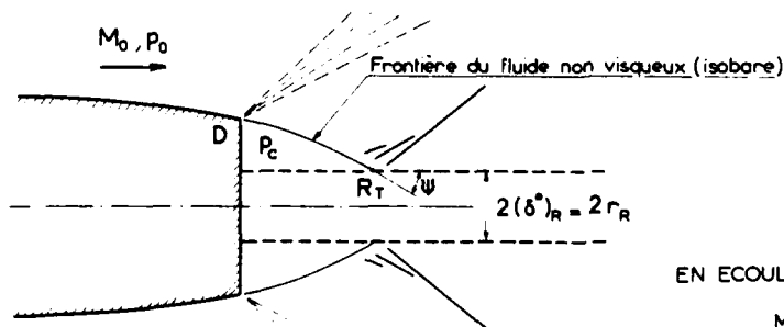
Fig. 67 - EFFET DE \gamma SUR LA PRESSION DE CULOT - THEORIE de MUELLER
