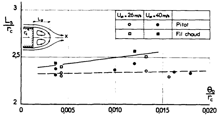
Fig. 7 EFFET DE LA COUCHE LIMITE INITIALE SUR LA LONGUEUR DE LA ZONE DE RECIRCULATION ECOULEMENT INCOMPRESSIBLE (d'après [ 11 ])
