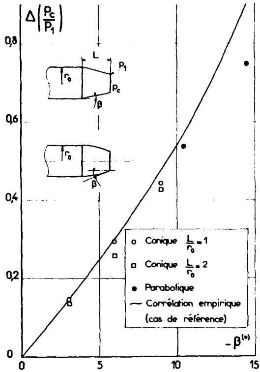
Fig. 18 EFFET DE RETREINT SUR LA PRESSION DE CULOT ECOULEMENT SUPERSONIQUE A M_0=2 (d'après [19.2])
