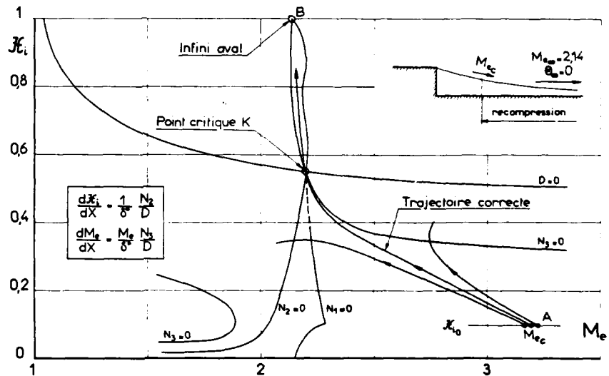
Fig. 63.- METHODE INTEGRALE TRAJECTOIRE DE LA SOLUTION DANS LE PLAN DE PHASE
