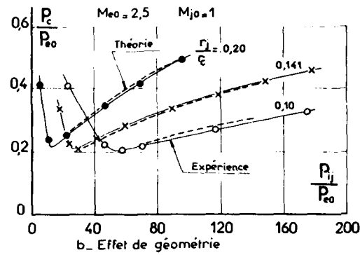
Fig. 93. CONFLUENCE EN AVAL D'UN CULOT - THEORIE D'ADDY
