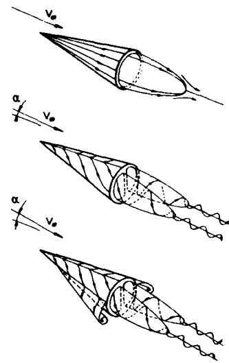
Fig. 23 EFFET D'INCIDENCE SUR LA STRUCTURE DE L'ECOULEMENT DE CULOT EN ECOULEMENT SUPERSONIQUE (d'après [ 23 ])
