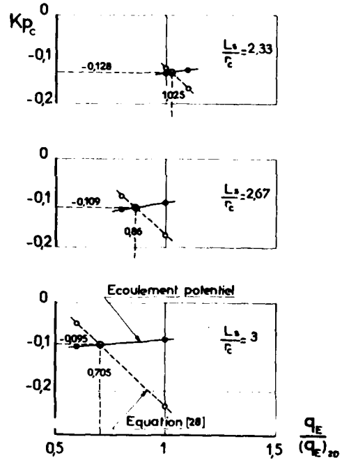
Fig. 79 - DETERMINATION DU DEBIT q_E (THEORIE de VANWAGENEN)
