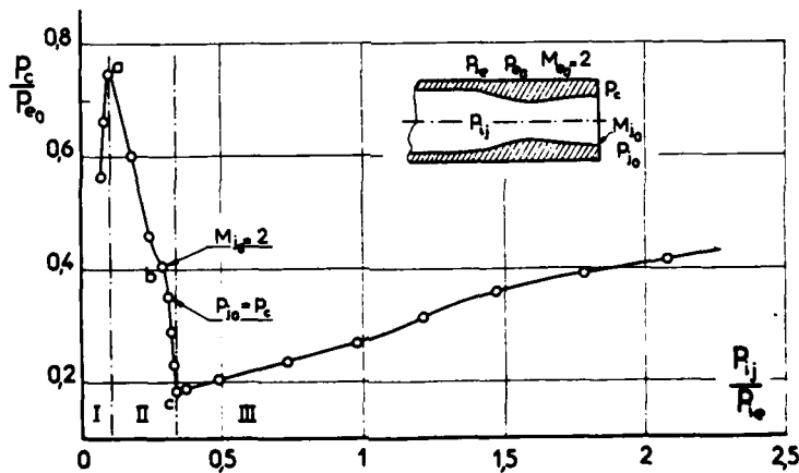
Fig. 31 PRESSION AU CULOT D'UN ARRIERE-CORPS EQUIPE D'UNE TUYERE EN ECOULEMENT SUPERSONIQUE (d'après [27])
