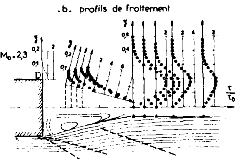
Fig. 13 STRUCTURE DE L'ECOULEMENT AU CULOT D'UN ARRIERE-CORPS CYLINDRIQUE ECOULEMENT SUPERSONIQUE ( d'après [ 15 ] )
