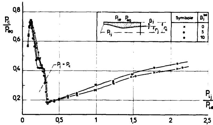
Fig. 37 EFFET DE L'ANGLE DE DIVERGENCE DE LA TUYERE SUR LA PRESSION DE CULOT (d'après [27])
