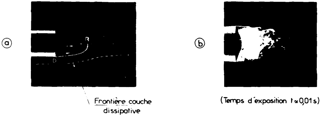
Fig. 2 ECOULEMENT DE CULOT VISUALISE AU TUNNEL HYDRODYNAMIQUE (d'après [ 10 ])
