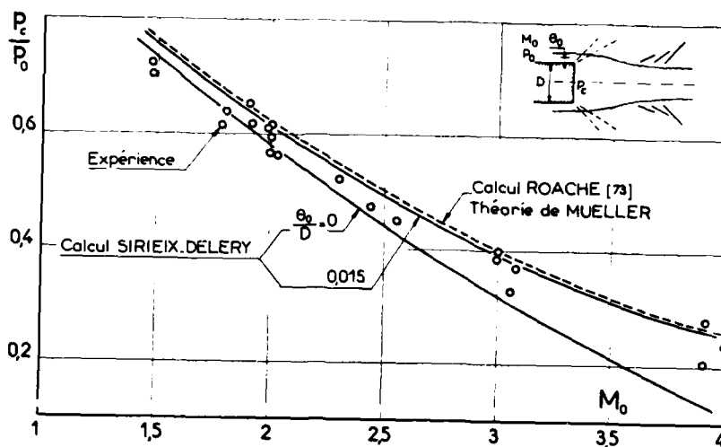
Fig. 69 - COMPARAISON CALCUL-EXPERIENCE THEORIES de SIRIEIX DELEERY et de MUELLER
