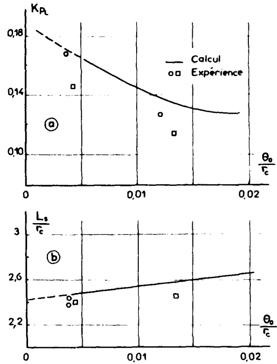
Fig. 82 COEFFICIENT DE PRESSION AU RECOLLEMENT ET LONGUEUR DE CAVITE (THEORIE de VANWAGENEN)
