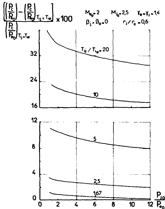
Fig. 98 VARIATION PARAMETRIQUE DE \frac{T_{ij}}{T_{ie}} (d'après ADDY [90])
