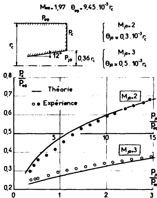
Fig 85 RECOLLEMENT SUR PAROI ET RECOLLEMENT SUR UNE NAPPE FLUIDE
