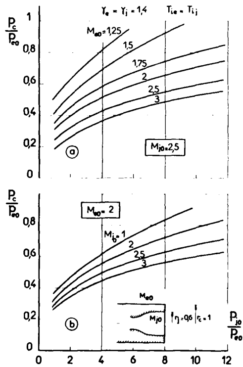
Fig. 95 VARIATION PARAMETRIQUE DE M_{00} (a) ET DE M_{j0} (b) (d'après ADDY [90])
