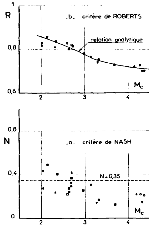
Fig. 56 - CRITERES DE RECOLLEMENT DE NASH ET DE ROBERTS
