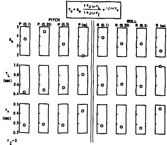
Fig. 7 Pilot model parameters
