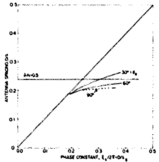
(d) Dipole length b = 0.420 m
