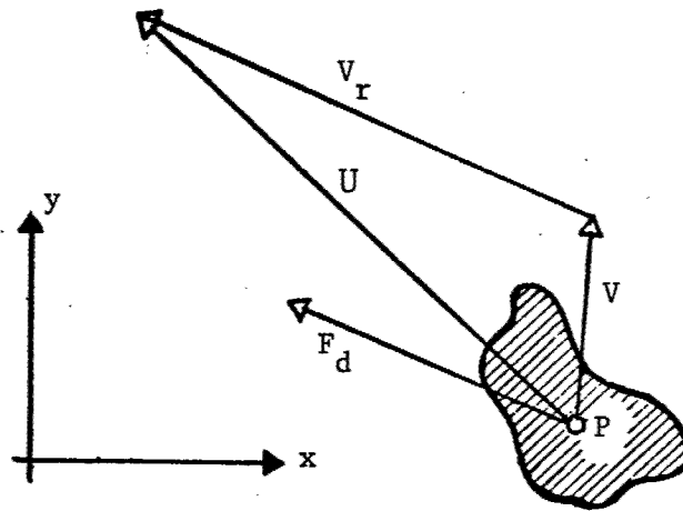
a) Simple Drag Model
