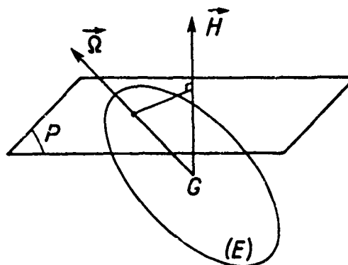
Fig. 6 - Mouvement d'Euler-Poinsot général.
