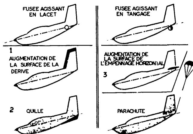
Fig. 6 - MODIFICATIONS ET DISPOSITIF
