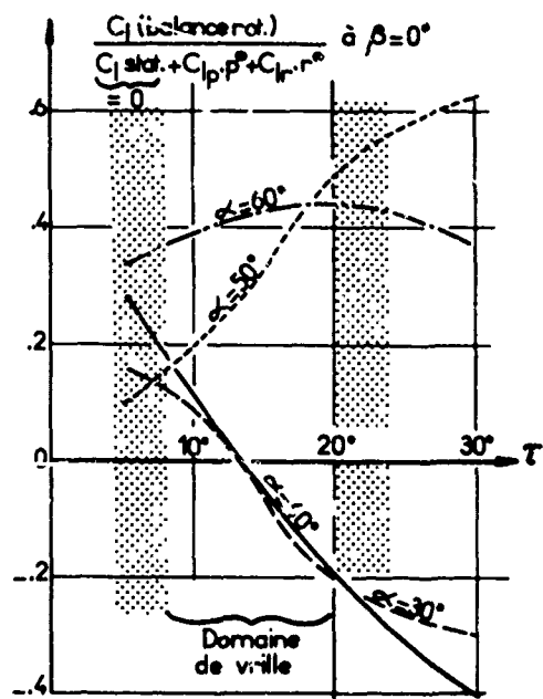
Fig. 14 - Rapport des C_l globaux mesuré et calculé.
