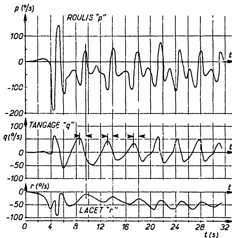
Fig. 5 - Vrille calculée du F5. réf Weissman ASD TR.72 48
