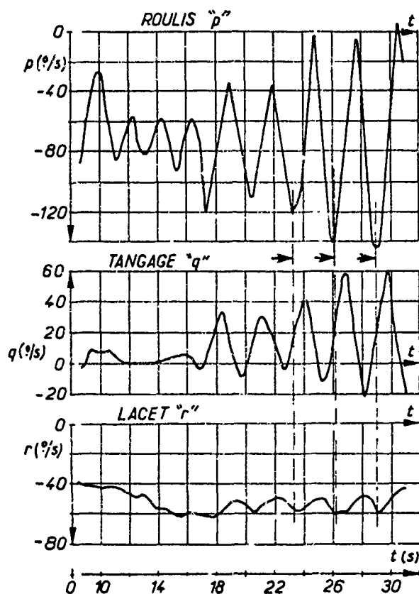
Fig. 3 - Vrille du Fouga CM 170. réf. Leconte, Mécanique du Vol, Dunod.
