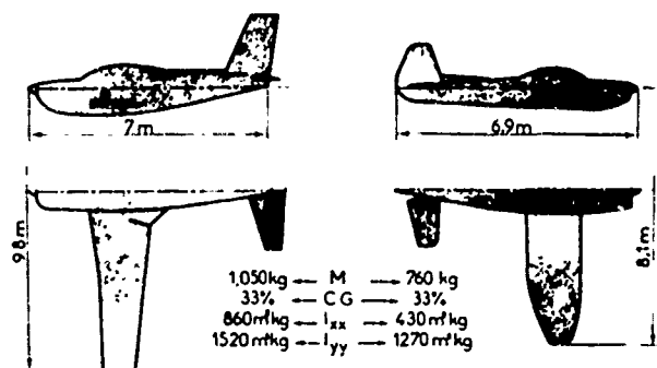
Fig. 1 - MAQUETTES UTILISEES (CARACTERISTIQUES DONNEES EN VALEUR AVION)
