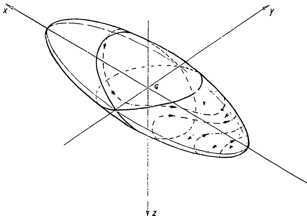
Fig. 15 - Sortie de vrille en autotonneaux.
