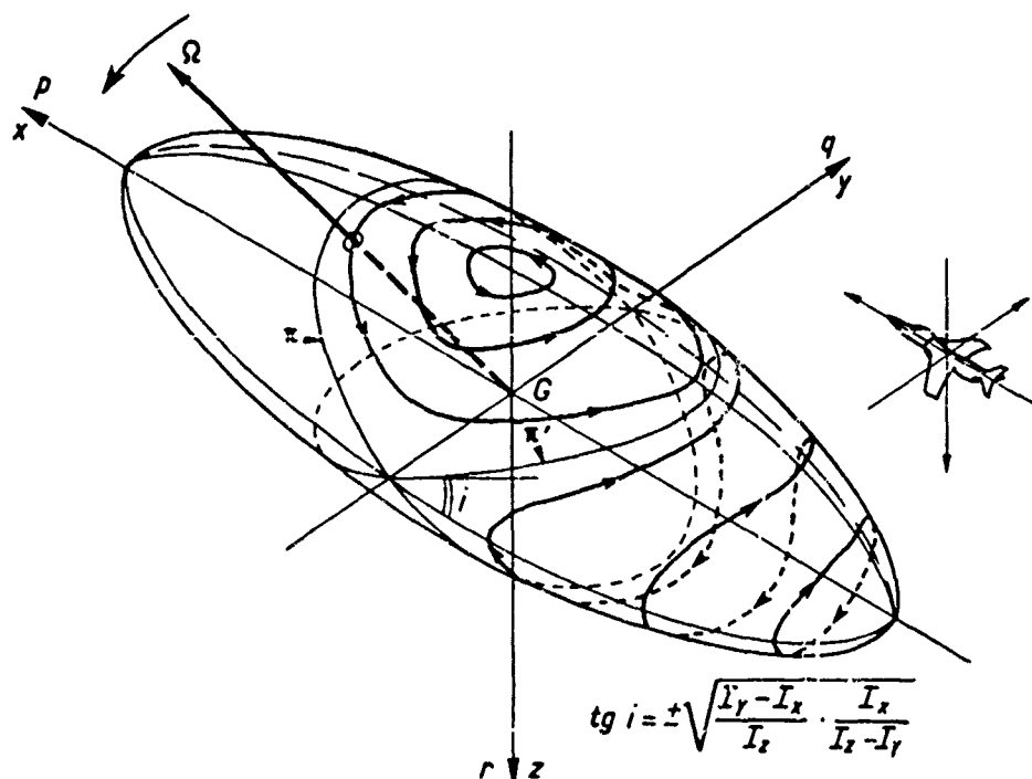
Fig. 7 - Mouvement d'Euler-Poinsot - Polhodies.
