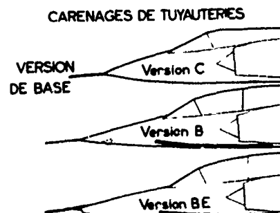
Fig. 23 - Différentes versions du Mirage Delta
