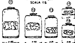
CARTOCCI A SACCHETTO PER CANNONI DA 49/35 SCALA 1:6
