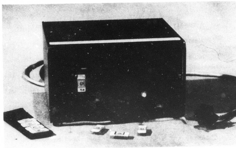
FIG. 3.2 ROM PROGRAMMER
