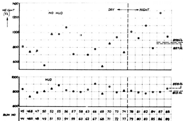
FIG. 5c: RANGE 5000 m.
