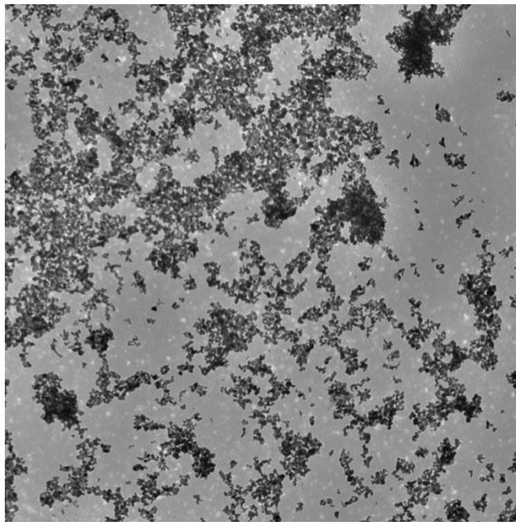
CEHR-24 05.tif CEHR-24 TiO 2 rutile 5-15 nm
