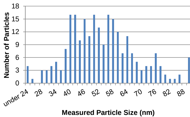
CEHR-26 02.tif CEHR-26 TiO 2 rutile 30-50 nm
