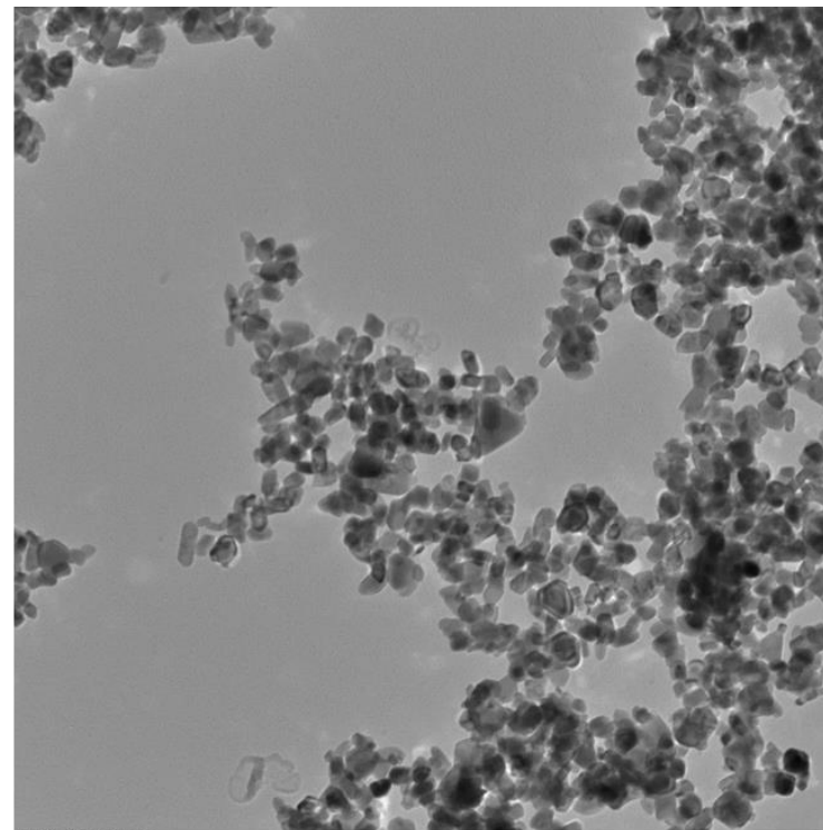
CEHR-26 04.tif CEHR-26 TiO 2 rutile 30-50 nm
