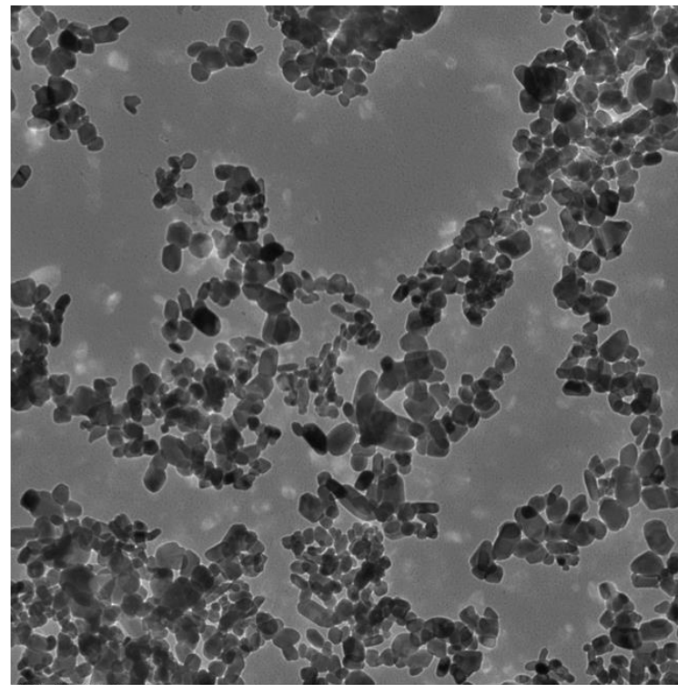
CEHR-24 06.tif CEHR-24 TiO 2 rutile 5-15 nm
