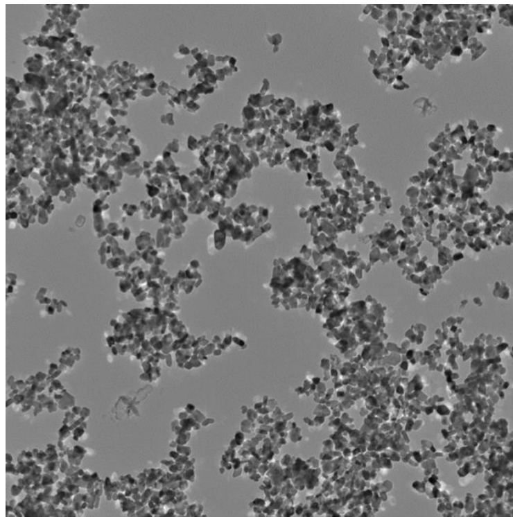
CEHR-26 02.tif CEHR-26 TiO 2 rutile 30-50 nm
