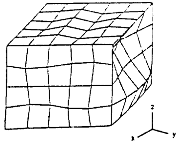
Mode 3 (1762 Hz)
