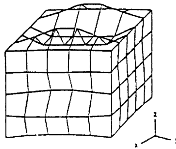
Mode 5 (2336 Hz)
