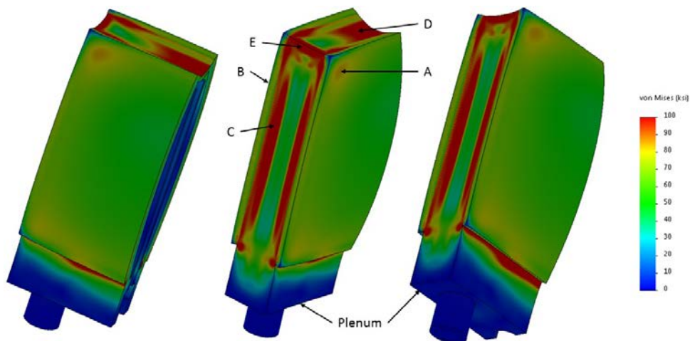
Fig. 12 MR 2.1.4 stress due to thermal load
