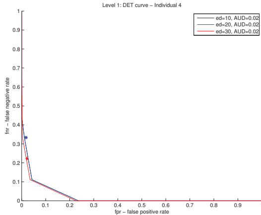
Fig. 4: DET curve.
