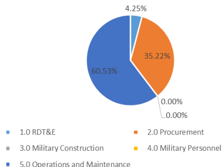
AMAS-ACO
