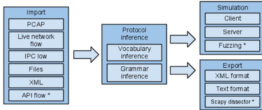
Fig. 1 Netzob main modules
