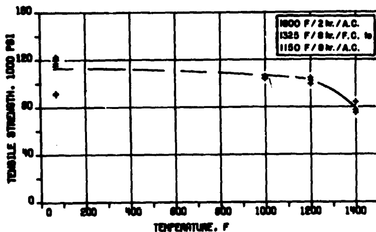
Tensile Strength
