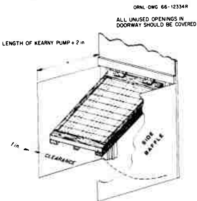
Fig. B-23. Side baffles.
