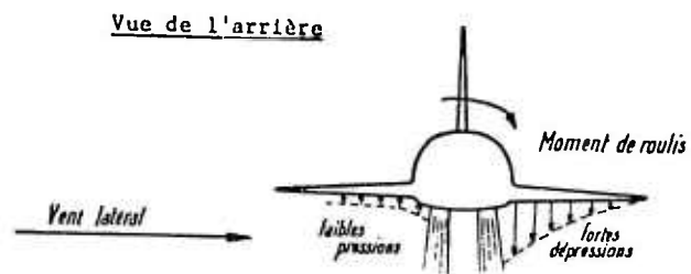
Fig. No. 3 Origine du moment de roulis -- dérapage positif dû aux jets des réacteurs verticaux
