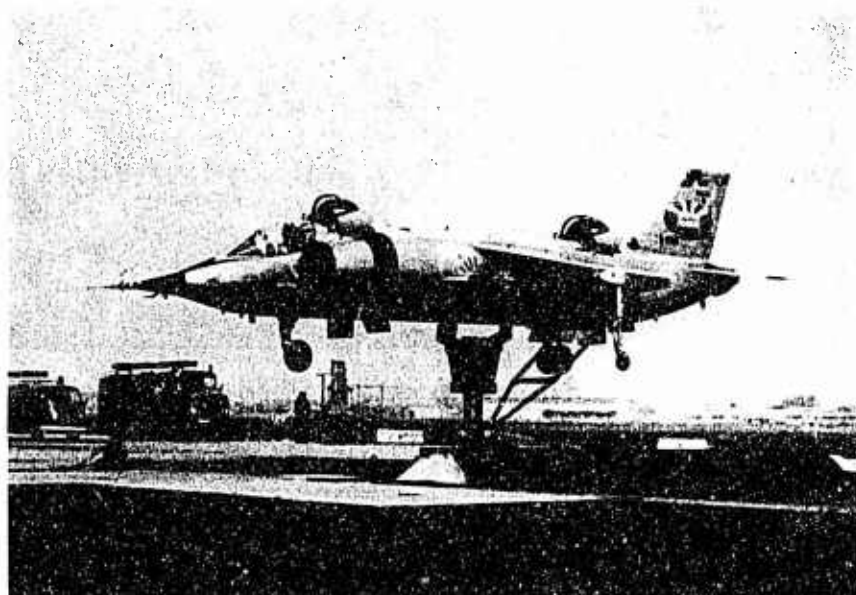
FIG. 11 VAK 191 B, TETHERED TEST
