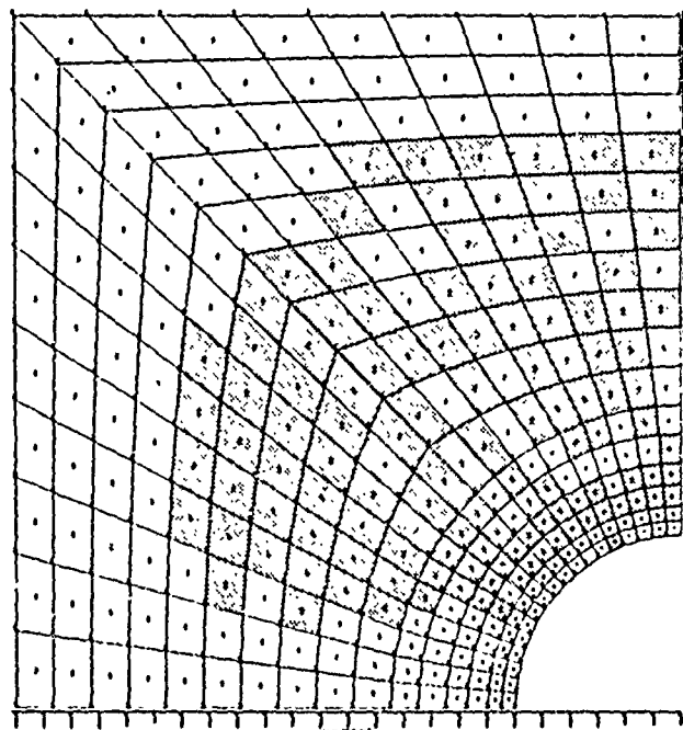
(d) LAST STEP OF GROUND SHOCK UNLOADING-- FIRST ATTACK
