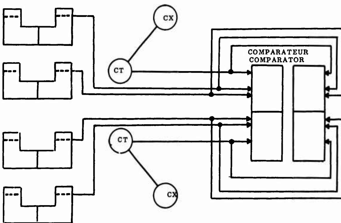
ELEVONS MEDIANS ET EXTERNES - MID AND OUTER ELEVONS
