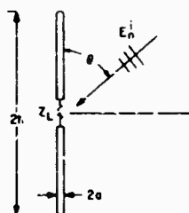
Fig. 1 - Linear antenna
