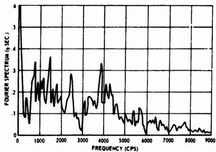
Fig. 20. Fourier amplitude spectrum-- test 2, accelerometer 9L
