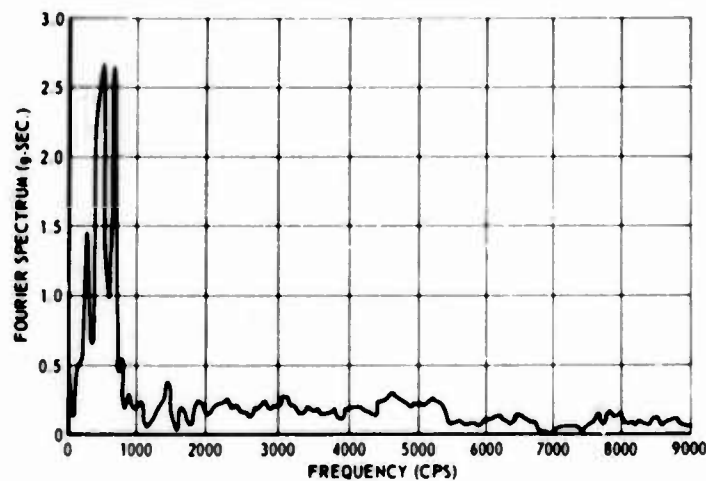
Fig. 17. Fourier amplitude spectrum -- test 2, accelerometer 1R
