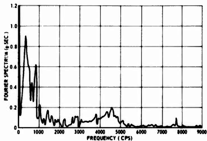
Fig. 21. Fourier amplitude spectrum-- test 2, accelerometer 9R
