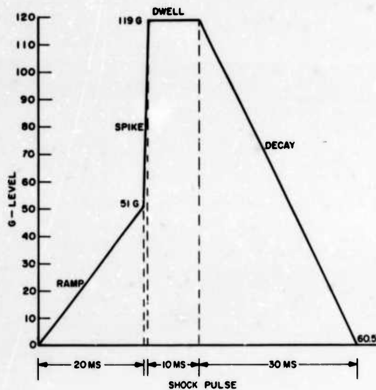
Fig. 1. Shock pulse
