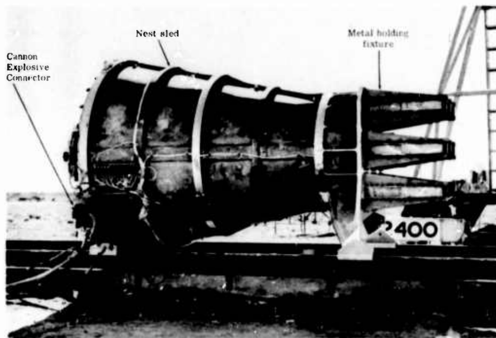
Fig. 12. Nest sled
