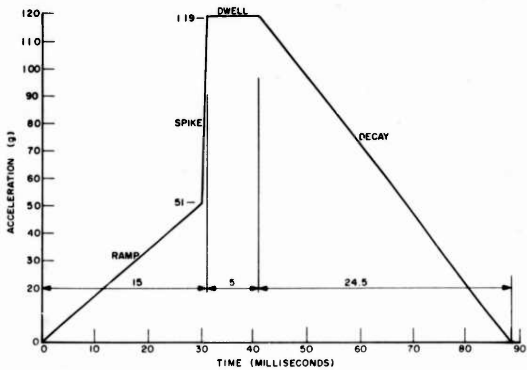
Fig. 11. Final input pulse
