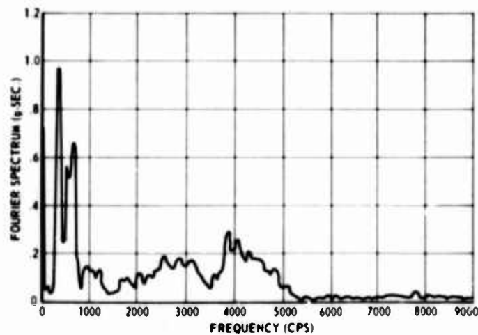
Fig. 18. Fourier amplitude spectrum -- test 2, accelerometer 6L
