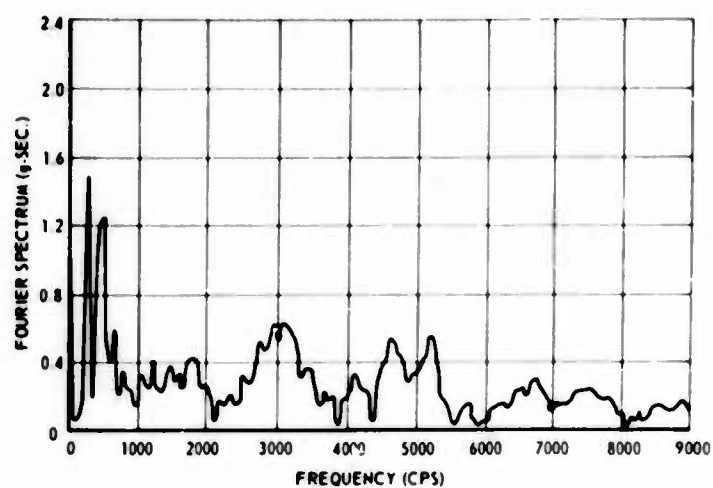
Fig. 16. Fourier amplitude spectrum -- test 2, accelerometer 1L
