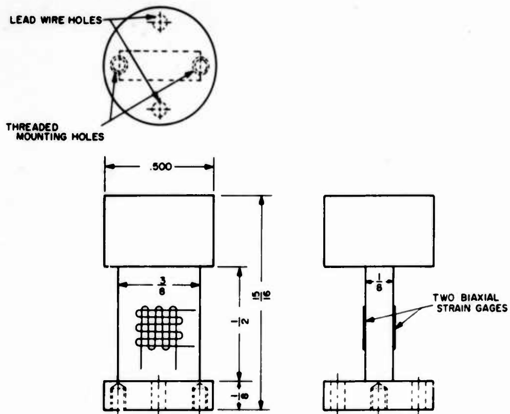
Fig. 4. Miniature load cell
