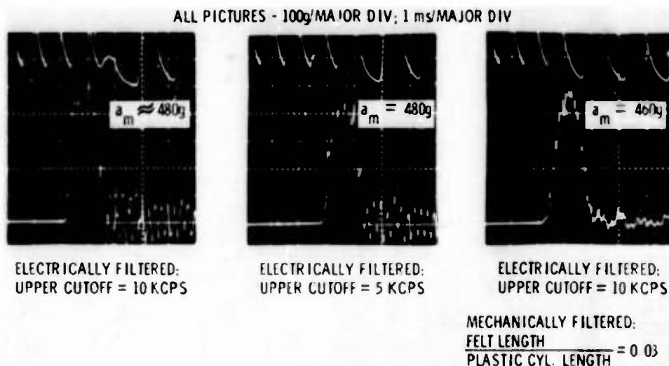
Fig. 7. Noisy pulse records
