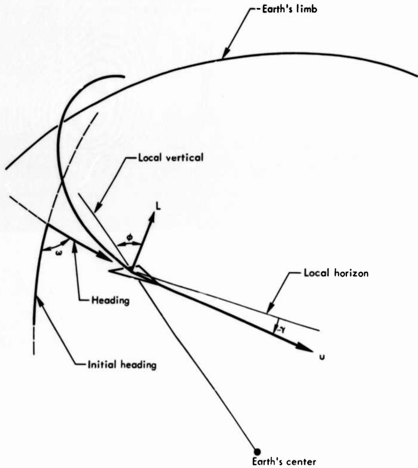
Fig. 1—Flight trajectory coordinates
