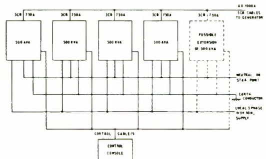
FIG. 7(a). 2000 kVA Resistance Load Bank.
