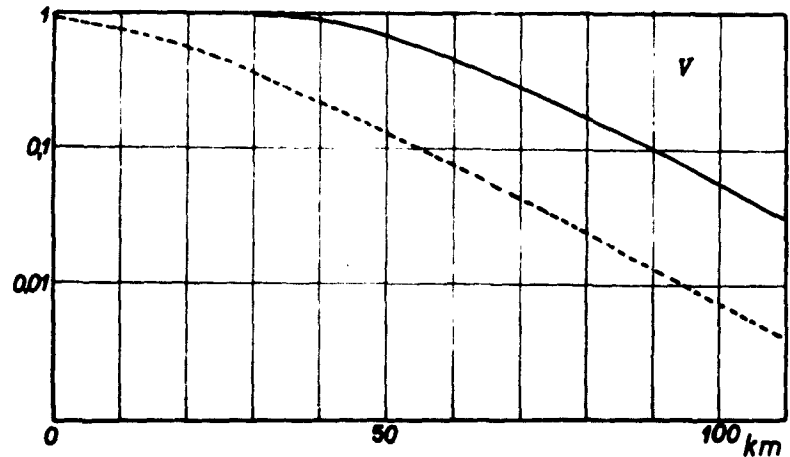
Fig. 5. — Luminance atmosphérique en fonction de l'altitude. Atmosphère polluée proportionnellement à la densité (cas V).
