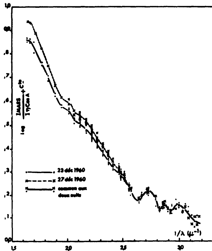
FIG. 1. Deux comparaisons de Mars à \eta Cas A.
