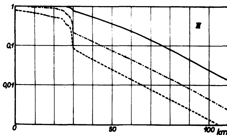
Fig. 3. — Luminance atmosphérique en fonction de l'altitude. Couche épaisse à l'altitude de 30 km (cas III) dans l'atmosphère pure.
