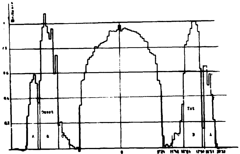
Fig. 7. — Saturne 9.VII.61 Coupe Photométrique W.E. corrigée de l'étalement. — Solution obtenue après 17 itérations.
