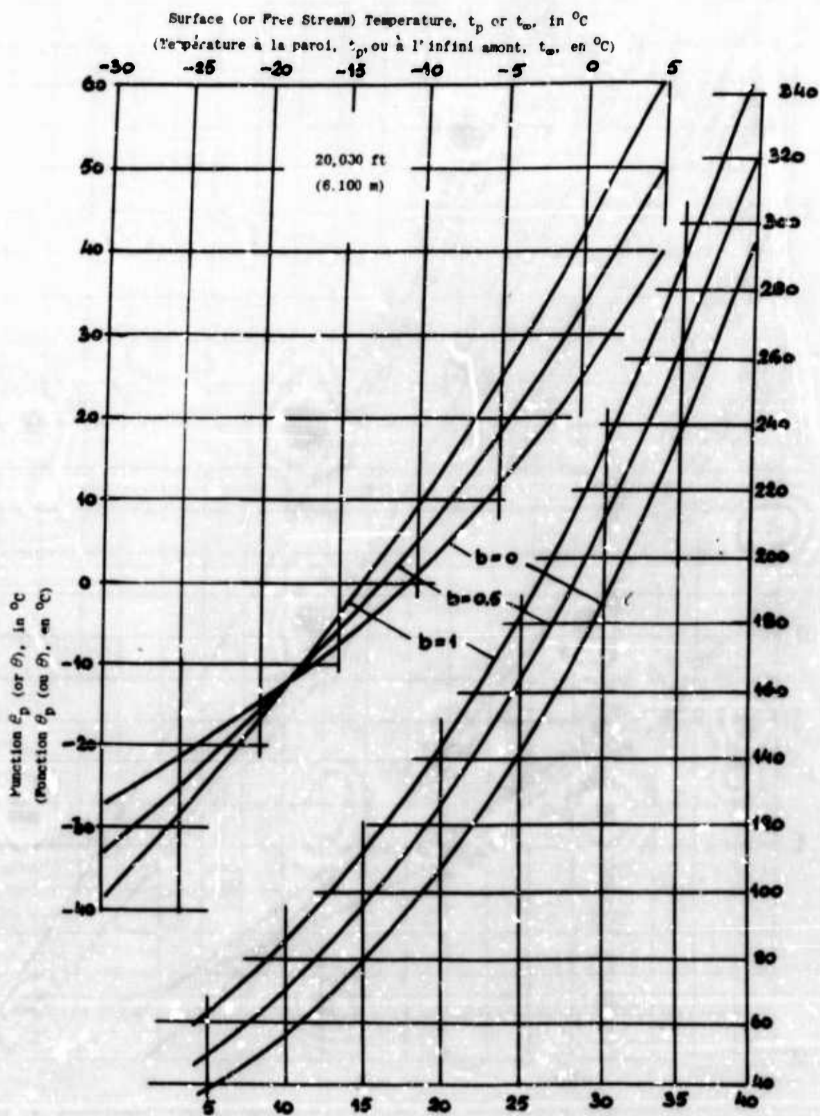
Fig. 16 Function \theta_p (or \theta ) versus t_p (or t_\infty ), for 20,000 ft altitude } (Ref. 46 Courbes de \theta_p (ou \theta ) en fonction de t_p (ou t_\infty ), à une altitude } Fig. 8) de 6.100m
