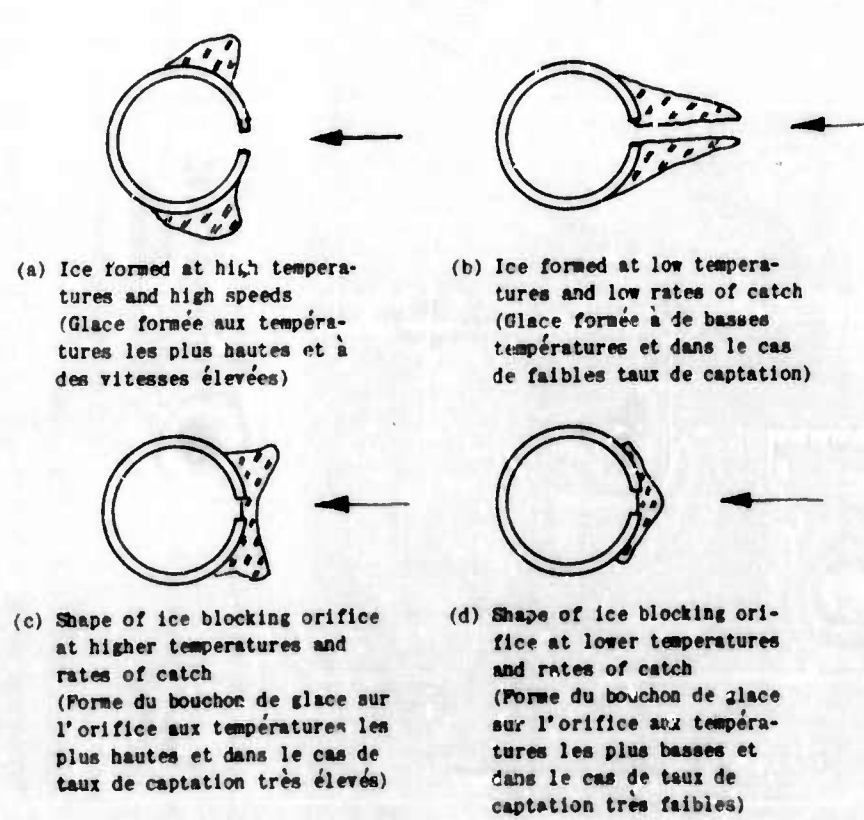
Fig. 12 Ice formations on orifice-type icing probe Formations de glace sur la sonde à orifices
