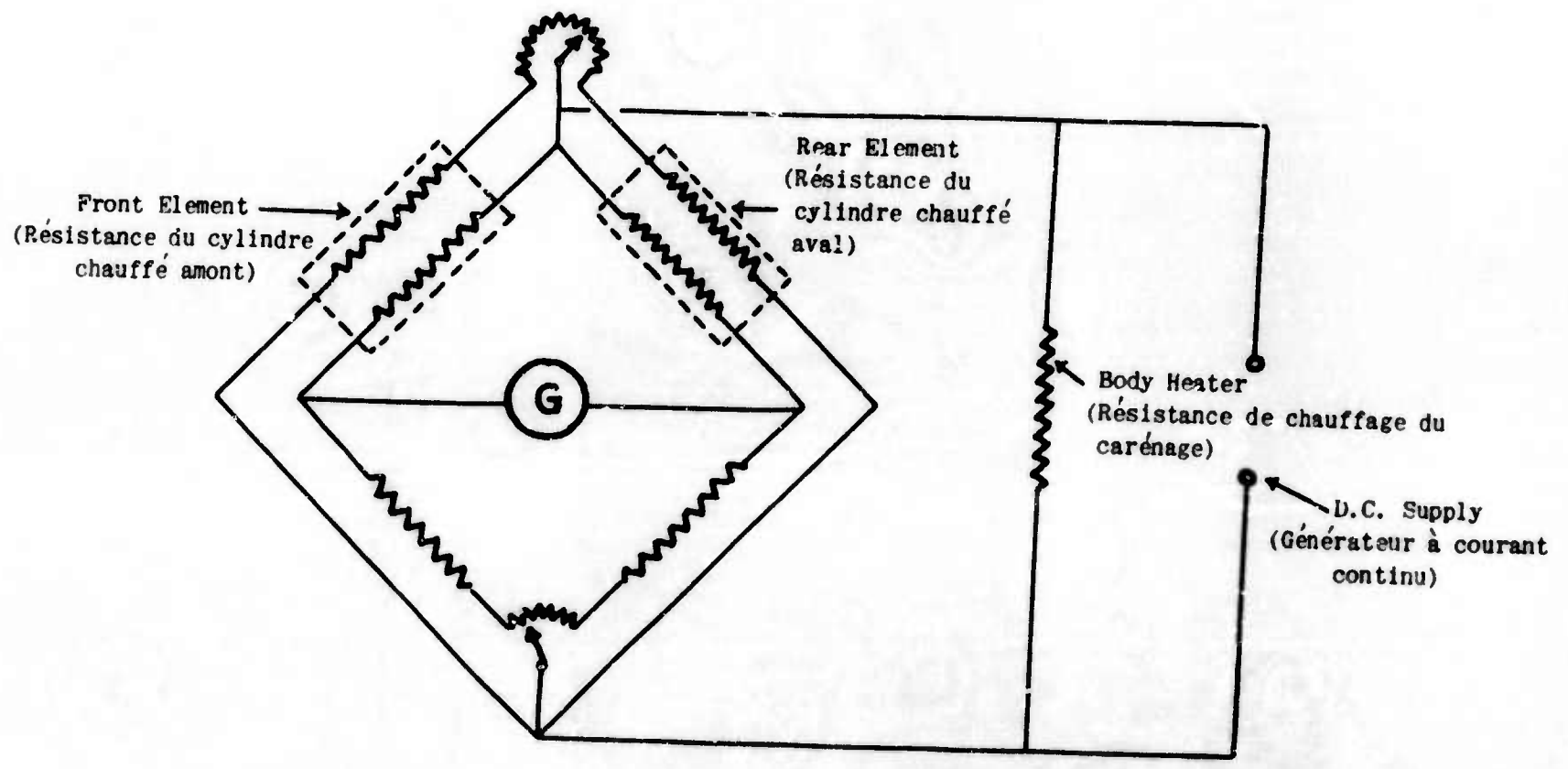
Fig. 8 Heated cylinders electrical circuit Circuit électrique de l'appareil à cylindres chauffés
