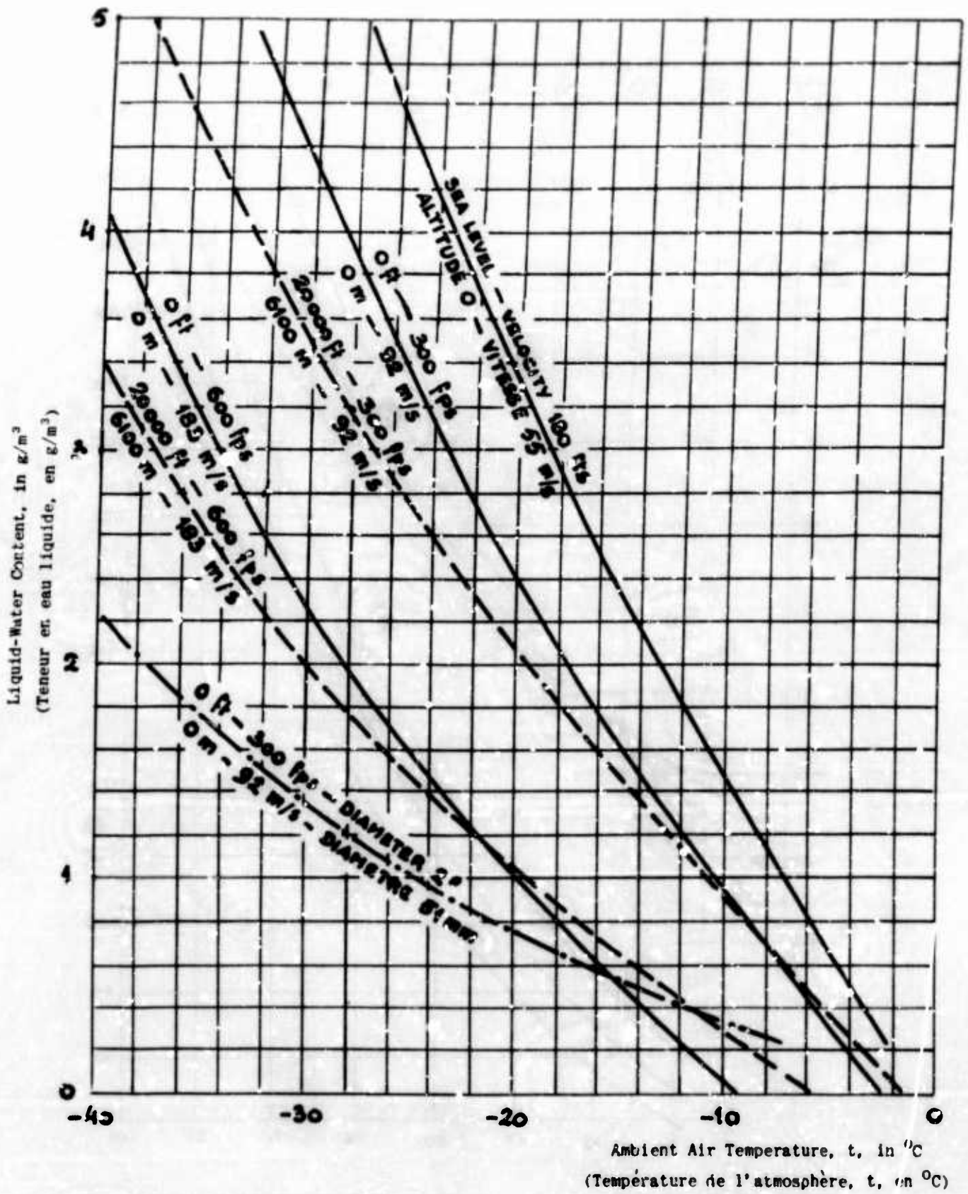
Fig. 17 Calculated Ludlam lines for 1/8 in. diameter rotating cylinder } (Ref. 48 Limites de congélation totale calculées pour un cylindre tournant } Fig. 1) de 0,32cm de diamètre
