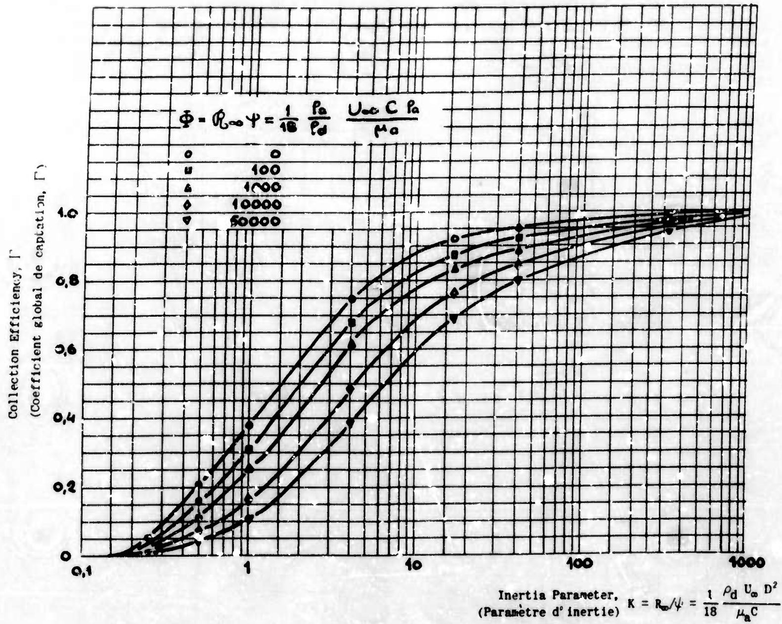
Fig. 11 Circular cylinder collection efficiency } (Ref. 16 Coefficient global de captation d'un cylindre circulaire } Fig. 7)
