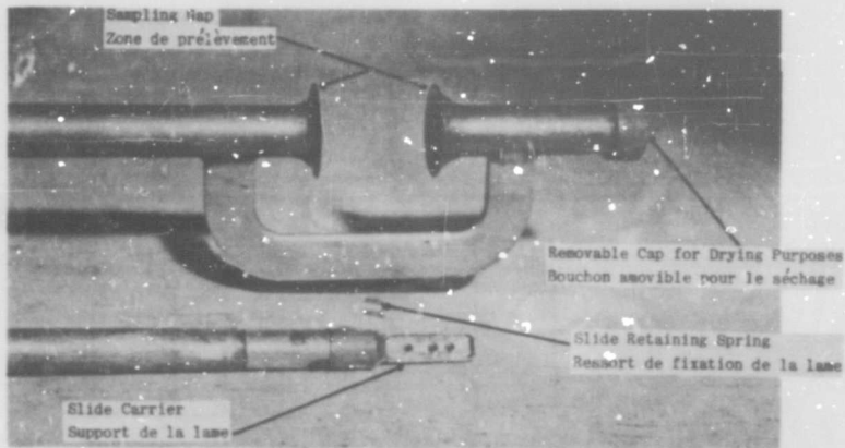
Fig. 20 Droplet sampling apparatus } (F.J. Bigg, R.A.E.) Appareil pour prélèvement de gouttelettes
