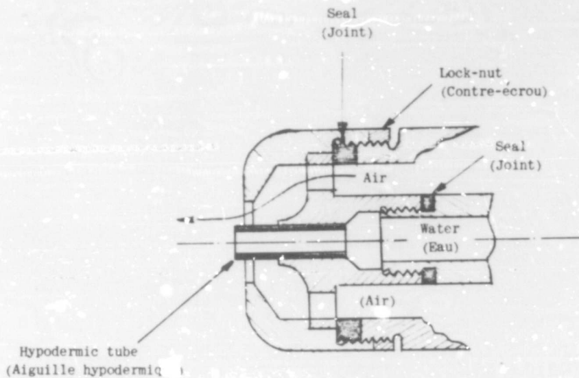
Fig. 19 RAE air blast atomiser - Pulvériscteur pneumatique RAE
