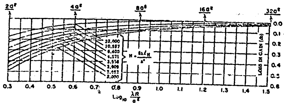
(b) H-plane
