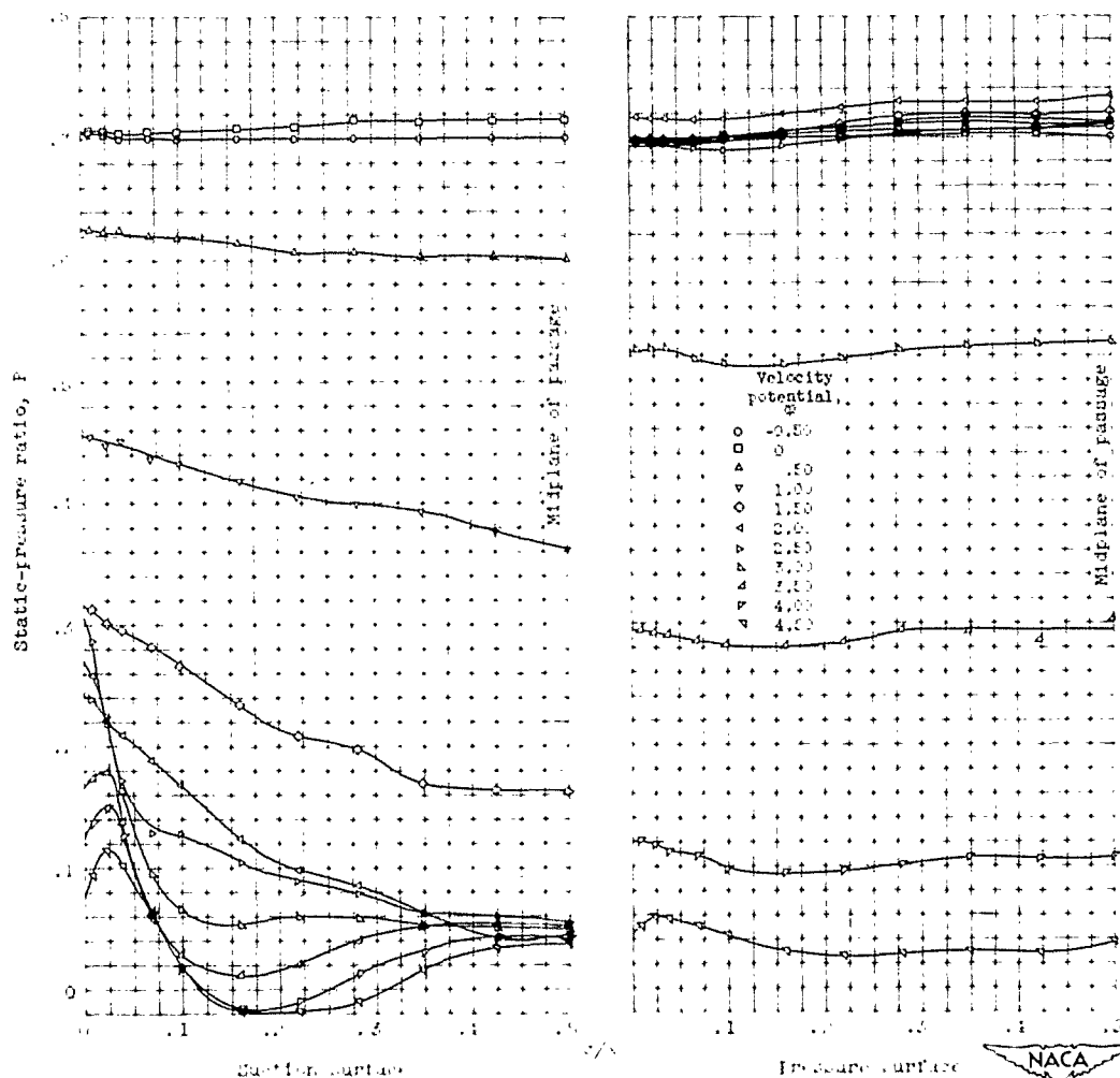
(d) 1.5-Inch spoiler.
