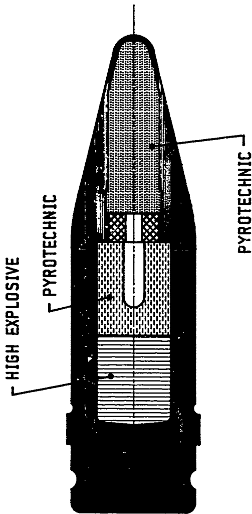
20mm PIÉ PROJECTILE
