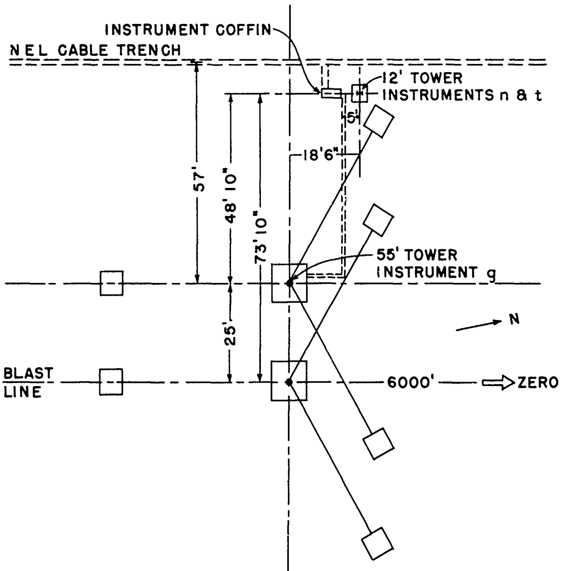
Fig. 2.10 7-208 Layout
