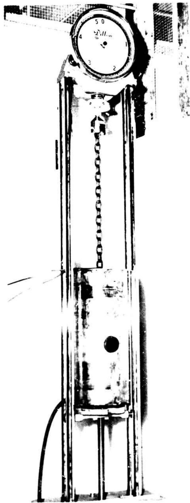
Fig. 6 Low-Temperature Tensile-Test Apparatus
