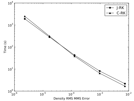
(d) FR time for given accuracy on Intel i3
