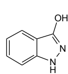
1H-indazol-3-ol
