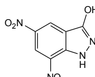
5,7-dinitro-1H-indazol-3-ol
