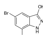
5,7-dibromo-1H-indazol-3-ol
