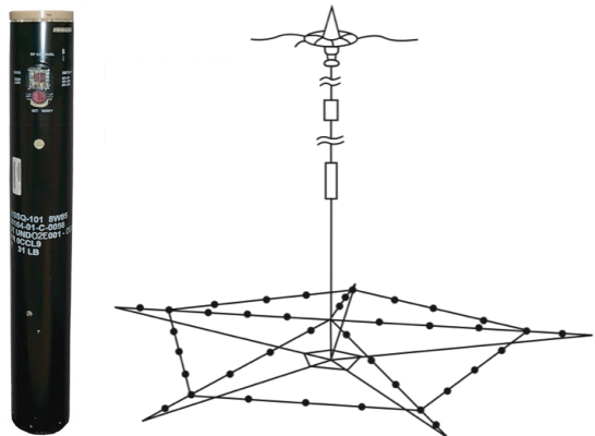
Fig. 4 – AN/SSQ-101 Sonobuoy
