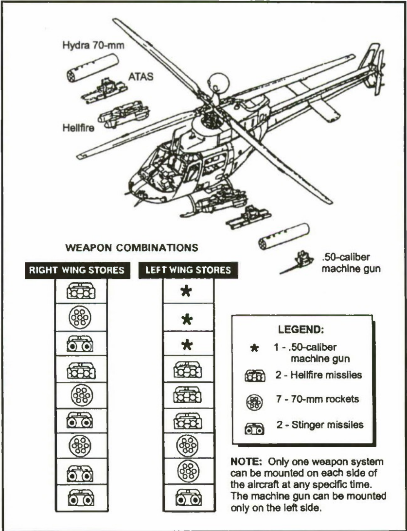
Figure 6-7. OH-58D(I) Kiowa Warrior.
