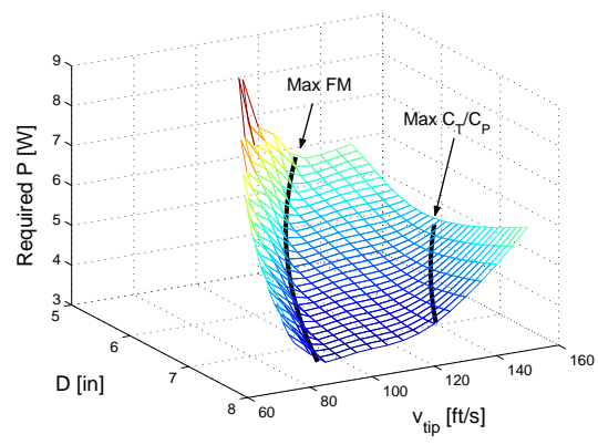
(d) Required power
