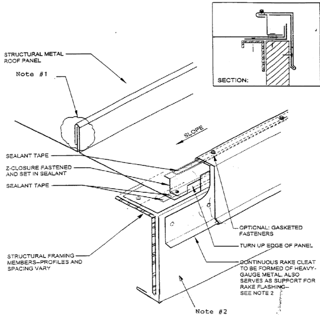
SVM-4 Rake Edge Flashing--End Panel
