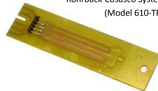
ER probe
