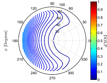
(d) DOLP of Fe, 2^{1/2}\sigma_h/\ell = 0.6 .
