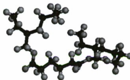
Polyazoture de glycidyle (GAP et GpI)
