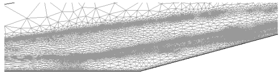
(d) Mesh, p = 3
