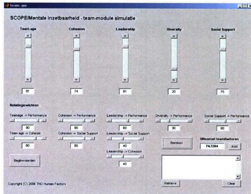
Figuur 3 Grafische interface van het experimentele computermodel in Matlab.
