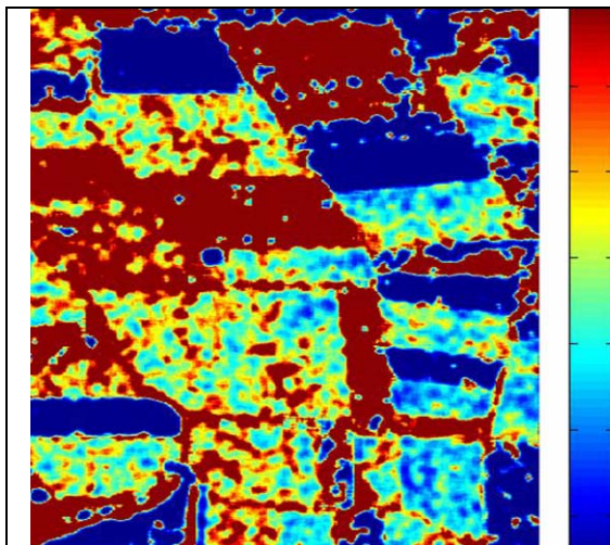
Fig. 10.3a Volumetric Soil Moisture Map mv [vol. %](Hajnsek et. al. 2000)
