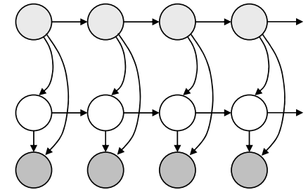
(d) Input-output HMM
