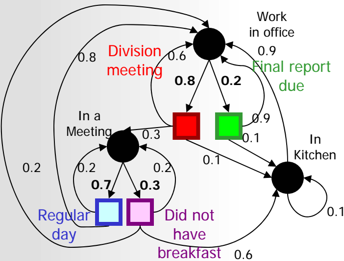
POMDP
