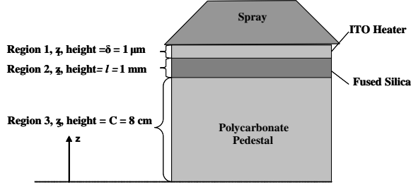
F i g A. n a l y t i c a l d o m a i n f o r h e a t e r a n d h e a t e r s u p p o r t s t r u
