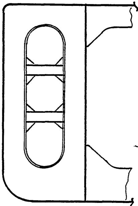
TANKER WEB FRAME
