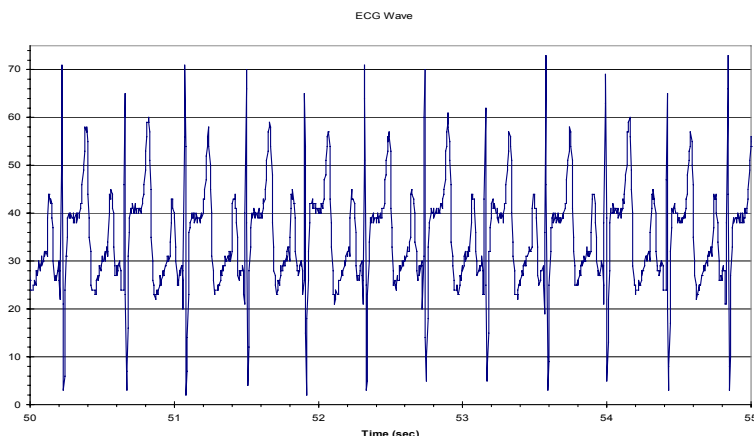
ECG 120-150 bpm
