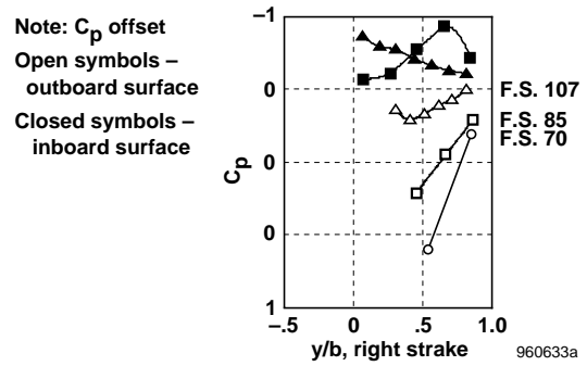
(d) \delta_{s,LR} = 0^\circ/90^\circ , M = 0.24 , Re_c = 9.4 \times 10^6 .
