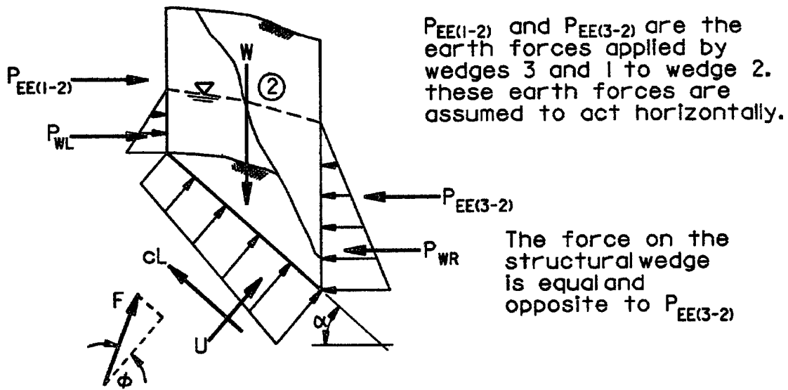
b. Free body of wedge 2
