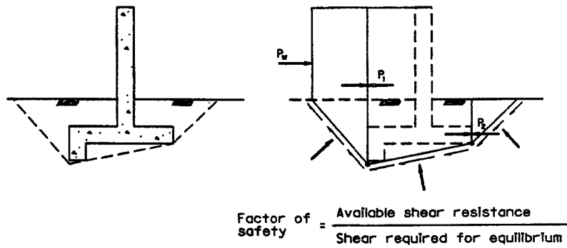
a. Sliding
