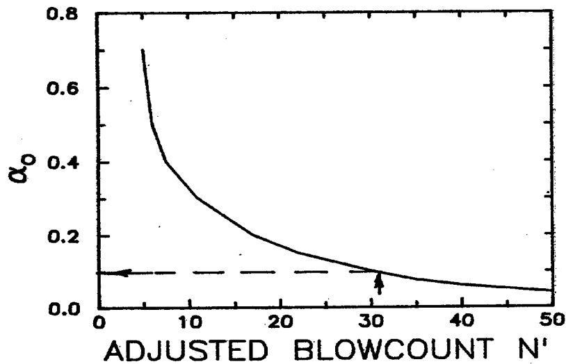
b. PARAMETER \alpha_0 FROM ADJUSTED BLOWCOUNT
