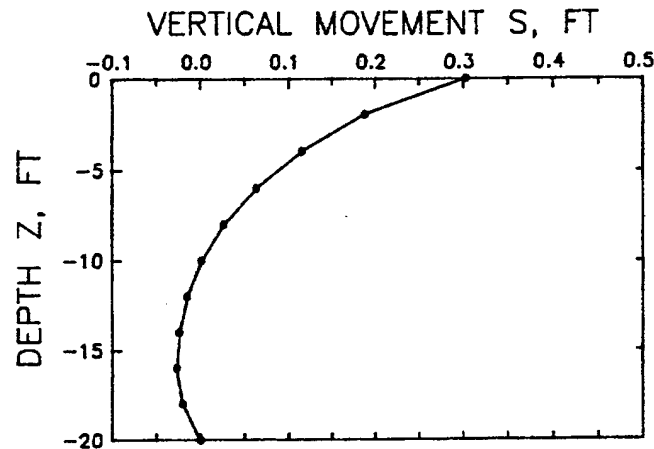
a. BENEATH SLAB
