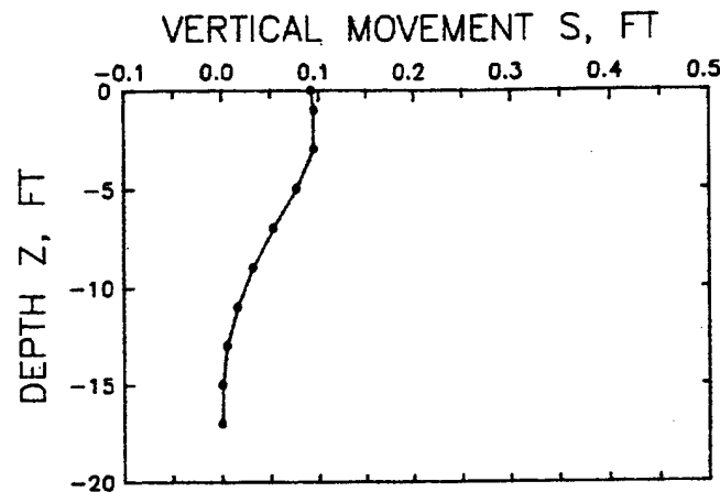
b. BENEATH COLUMN
